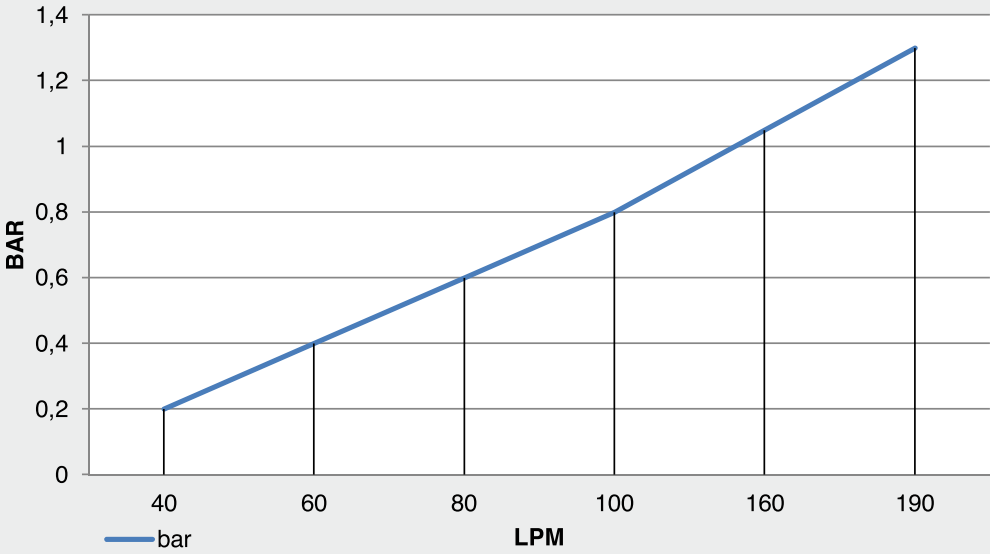
DIAGRAMMA PERDITE DI CARICO - PRESSURE DROP DIAGRAM
