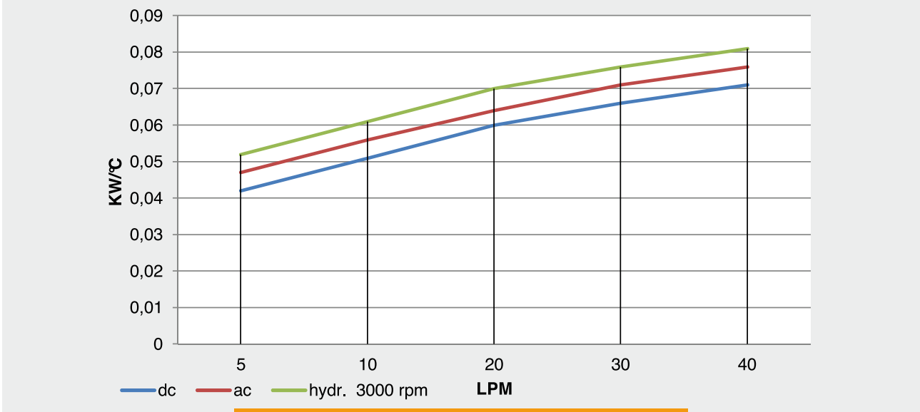
DIAGRAMMA DI RENDIMENTO - PERFORMANCE DIAGRAM
