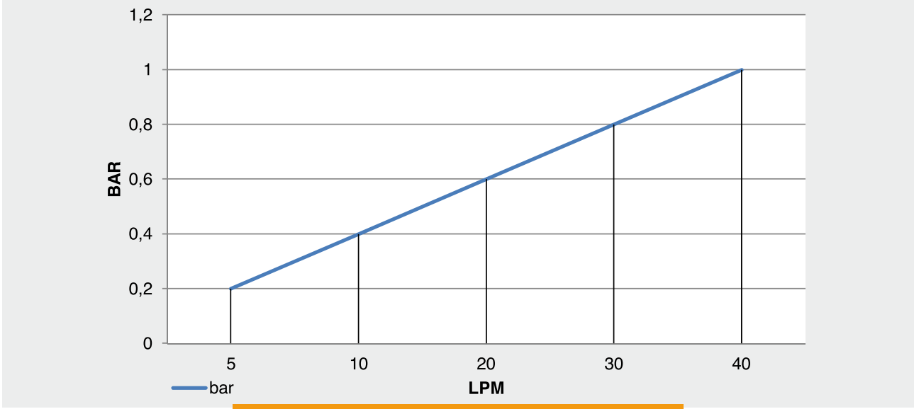
DIAGRAMMA PERDITE DI CARICO - PRESSURE DROP DIAGRAM
