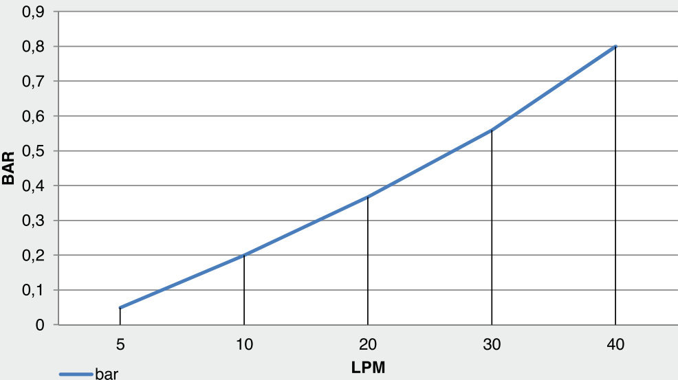
DIAGRAMMA PERDITE DI CARICO - PRESSURE DROP DIAGRAM
